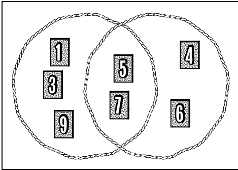
Рис. 47. Пересекающиеся множества.
