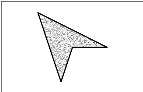
Рис. 52. Невыпуклый четырёхугольник.
