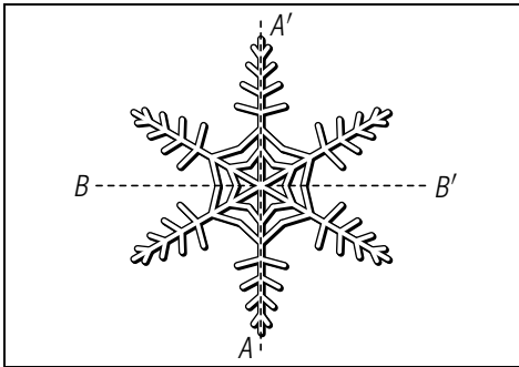
Рис. 67. Симметрии снежинки.
