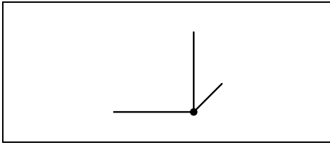
Рис. 156. Вершина куба.
