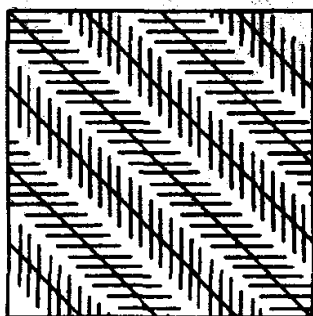
ИЛЛЮЗИЯ ЦЕЛЬНЕРА
