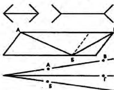
ИЛЛЮЗИИ МЮЛЛЕР-ЛИЕРА
