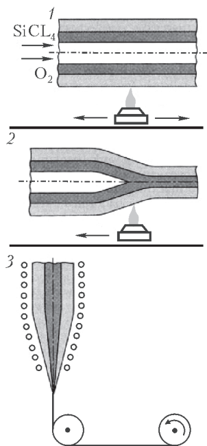
Рис.127. Основные этапы изготовления кварцевого волокна: 1 – осаждение кварца на внутренней поверхности кварцевой трубки при ее нагреве; 2 – «схлопывание» трубки при дальнейшем ее нагревании; 3 – вытяжка кварцевого волокна с диаметром 10\text{--}100\text{ мкм} и наматывание его на катушку
