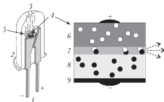
Рис.8. Светодиод в разрезе (слева) и строение полупроводникового чипа, испускающего свет (справа): 1 – металлические контакты для подключения к источнику постоянного тока; 2 – прозрачный кожух светодиода; 3 – свет, испускаемый светодиодом; 4 – полупроводниковый чип, слои которого схематически показаны справа; 5 – параболический зеркальный отражатель, собирающий свет в параллельный пучок; 6 – слой, обладающий «дырочной», или p-проводимостью; 7 – активный слой, химический состав которого определяет параметры испускаемого света; 8 – слой, обладающий «электронной», или n-проводимостью; 9 – электропроводящая подложка чипа. Электроны на схеме справа обозначены черными кружками, а «дырки» – белыми. Электрическое напряжение, приложенное между n- и p-слоями полупроводникового чипа, приводит к движению электронов из n-слоя (8) в активный слой (7). Одновременно туда же под действием приложенного напряжения движутся «дырки» из p-слоя (6). В активном слое «дырки» и электроны встречаются и уничтожают друг с другом, и при этом часть энергии выделяется в виде света (пунктирные стрелки)
