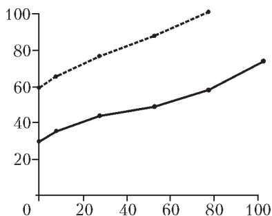
Рис. 110. Зависимость времени ожидания лифта (вертикальная ось, в секундах) от доли жильцов (горизонтальная ось, в %), вызывающих сразу оба лифта. Верхняя кривая – для тех, кто вызывает только один лифт, нижняя – для вызывающих оба лифта
