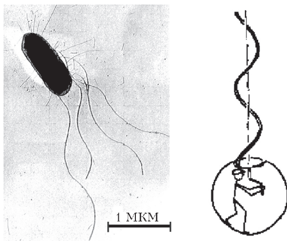
Рис.58. Фото бактерии кишечной палочки и схематическое изображение принципа ее движения с помощью закручивания жгутика
