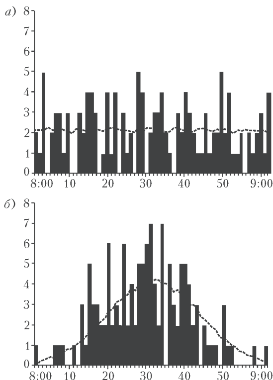
Рис.108. Зависимость количества жильцов (вертикальная ось), выходящих на лифтовые площадки 17-этажного дома каждую минуту, от времени между 8:00 и 9:00 утра (горизонтальная ось, в минутах). Черные столбцы – пример для одного из 365 дней года, пунктирная кривая – усредненное по 365 дням значение. Время выхода жильцов на лифтовые площадки задавалось генератором случайных чисел компьютера, предполагая их равномерное распределение (а) или нормальное распределение (б). С каждого этажа в течение этого часа лифт вызывают 8 человек
