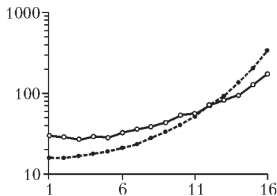
Рис. 112. Зависимость времени ожидания лифта (вертикальная ось, в секундах) от номера этажа (горизонтальная ось), с которого он вызван. Верхняя (более пологая) кривая – все жильцы вызывают один лифт, нижняя – все вызывают оба лифта
