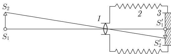
Рис. 244. Схема фотоаппарата: 1 — объектив, 2 — камера, 3 — фотопластинка
