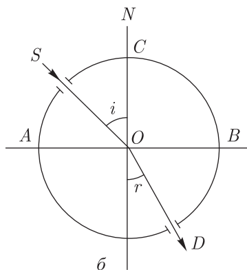
Рис. 181. Измерение угла отражения (а) и преломления (б)
