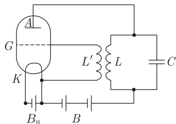
Рис. 58. Ламповый генератор
