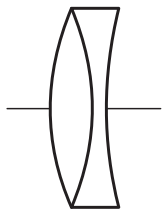
Рис. 233. Склеенный астрономический объектив, исправленный на сферическую aberrацию
