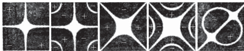
Рис. 103. Примеры фигур Хладни. Знаком плюс отмечены те пучности, где пластинка выгнута в данный момент вверх, а знаком минус — книзу. Через четверть периода пластинка сделается плоской, а еще через четверть периода плюсы прогнутся вниз, а минусы — вверх
