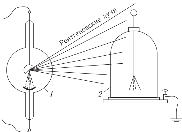
Рис. 303. Ионизирующее действие рентгеновских лучей: 1 — рентгеновская трубка, 2 — электроскоп. Опыт удастся как с положительно, так и отрицательно заряженным электроскопом. Под действием рентгеновских лучей в воздухе создаются ионы обоих знаков
