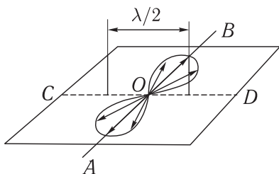
Рис. 121. Двойная синфазная антенна сильно излучает по направлениям OA и OB и не излучает по направлениям OC и OD
