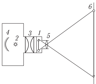
Рис. 240. Схема проекционного аппарата для демонстрации прозрачных объектов: 1 — объект, 2 — источник света, 3 — конденсор, 4 — вогнутое зеркало, 5 — объектив, 6 — экран
