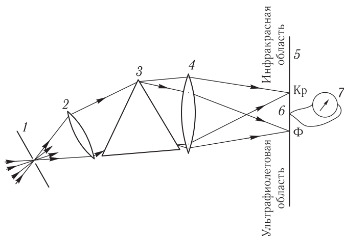
Рис. 297. Схема опыта по исследованию распределения энергии в спектре: 1, 2, 3, 4 — части спектрального аппарата, дающего спектр источника в плоскости 5, 6 — термоэлемент, могущий перемещаться вдоль спектра, 7 — гальванометр, Ф — фиолетовая граница спектра, Кр — красная граница спектра
