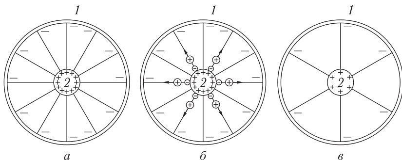
Рис. 385. К механизму работы газоразрядного счетчика частиц (1 — цилиндр счетчика, 2 — нить, диаметр которой преувеличен): а) счетчик заряжен до рабочей разности потенциалов, при которой прохождение заряженной частицы через счетчик вызывает в нем вспышку газового разряда. Изображены линии электрического поля в счетчике. Густота линий, т.е. напряженность электрического поля, наибольшая у нити; б) поле в счетчике в момент самогашения разряда. Электроны, образованные при ионизации газа, собрались на нити и компенсируют часть ее положительного заряда. Положительные ионы продолжают двигаться к цилиндру. Поле у нити ослаблено; в) поле в счетчике, не присоединенном к батарее, после того как разряд погас и положительные ионы дошли до цилиндра
