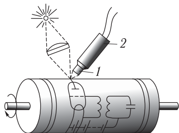
Рис. 146. Схема передающего устройства фототелеграфа: 1 — объектив, 2 — фотоэлемент
