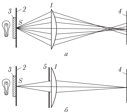
Рис. 228. Экспериментальное изучение сферической абберации: а) линза, на которую падает широкий пучок, дает расплывчатое изображение; б) центральная зона линзы дает хорошее резкое изображение
