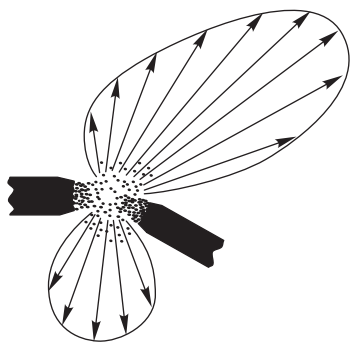
Рис. 160. Яркость электрической дуги, пропорциональная длине стрелок на рисунке, зависит от направления излучения
