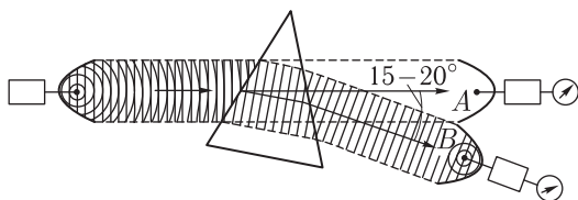
Рис. 131. Преломление электромагнитной волны в призме
