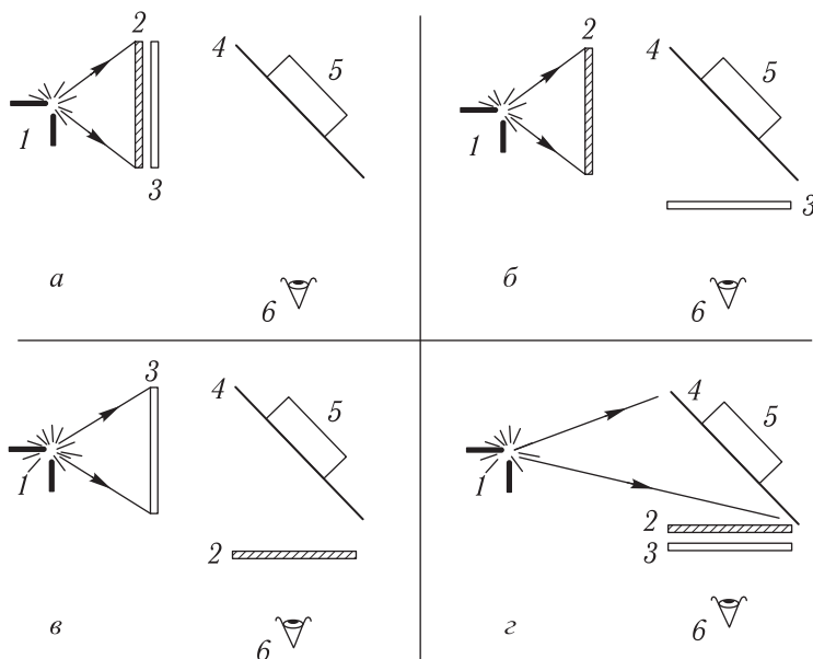
Рис. 347. К упражнению 40: 1 — дуга, 2 — фиолетовый фильтр, 3 — желто-зеленый фильтр, 4 — лист бумаги, 5 — сосуд с флуоресцеином, 6 — глаз
