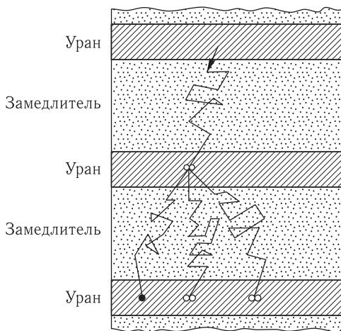
Рис. 407. Развитие цепной реакции деления в системе из природного урана и замедлителя. Быстрый нейтрон, вылетев из тонкого стержня, попадает в замедлитель и замедляется. Попадая снова в уран, замедленный нейтрон скорее всего поглощается в ^{235}\text{U} , вызывая деление (обозначение: два светлых кружка). Некоторые нейтроны поглощаются в ^{238}\text{U} , не вызывая деления (обозначение: черный кружок)
