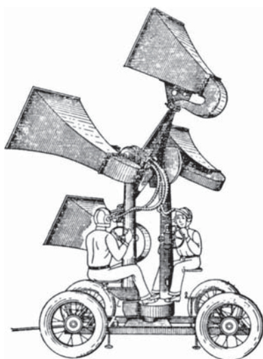
Рис. 113. Звукоулавливающая установка
