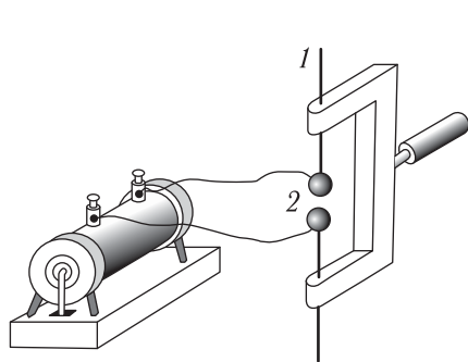
Рис. 122. Схема вибратора Герца
