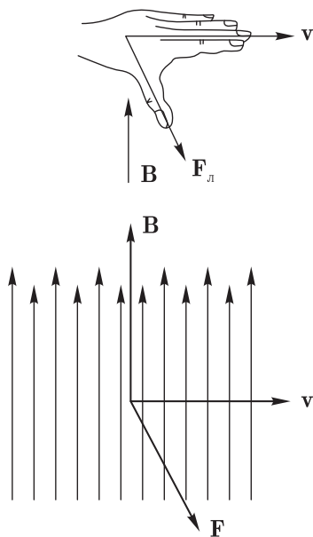
Рис. 349. Направление силы Лоренца \mathbf{F}_\text{л} , действующей на заряд, движущийся в магнитном поле \mathbf{B} со скоростью \mathbf{v} . Изображен случай положительного заряда. Для отрицательного заряда сила направлена в противоположную сторону
