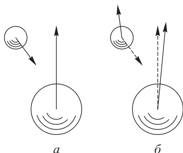
Рис. 357. Соударение тяжелого шара с легким. Сплошными стрелками показаны скорости шаров а ) до удара; б ) после удара; движение тяжелого шара изменяется в результате соударения незначительно (штриховые стрелки — скорости шаров до удара)
