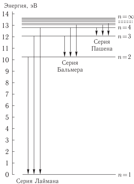
Рис. 360. Схема энергетических уровней атома водорода. Горизонтальные линии — энергетические уровни ( n — номер уровня). За начало отсчета по шкале энергий принята наименьшая внутренняя энергия атома водорода, т.е. энергия уровня n = 1 . Вертикальные линии — переходы с верхних энергетических уровней на нижние. Длина такой линии дает энергию h\nu светового кванта, излучаемого при данном переходе. Переходы группируются в серии: серия Лаймана — переходы с уровней n > 1 на уровень n = 1 , серия Бальмера — переходы с уровней n > 2 на уровень n = 2 и т. д. (см. также § 175)
