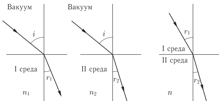
Рис. 184. Относительный показатель преломления двух сред:
