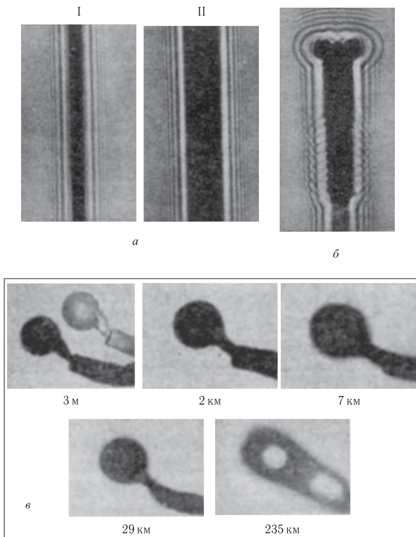
Рис. 275. Фотографии дифракционных картин (тень отбрасывается на экран): а) дифракция от проволоки (I) и карандаша (II); б) дифракция от шурупа; в) дифракция от руки, держащей тарелку, при различных расстояниях от руки до экрана
