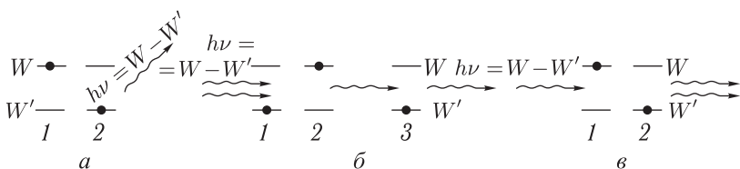
Рис. 361. а) Спонтанное излучение света: 1 — в результате столкновения с другим атомом или с электроном, или в результате поглощения светового кванта атом перешел на один из своих верхних уровней W (для простоты на схеме указаны только два квантовых уровня W и W' ), 2 — через некоторое время возбужденный атом сам по себе (без внешних воздействий) переходит на нижний уровень W' , испуская световой квант h\nu = W - W' . б) Резонансное поглощение света: 1 — атом, находящийся на уровне W' , облучается светом с частотой \nu = \frac{W - W'}{h} (резонансная частота), 2 — атом поглощает из светового пучка один квант h\nu = W - W' и переходит на уровень W ; световой пучок ослабляется; 3 — возбужденный атом при столкновении с другим атомом отдает ему энергию и возвращается на уровень W' (он может вернуться на уровень W' или перейти на другой уровень, расположенный ниже уровня W , также и путем излучения светового кванта). в) Вынужденное излучение света: 1 — атом, находящийся на верхнем уровне W , облучается светом резонансной частоты, 2 — атом испускает квант h\nu = W - W' в направлении падающего светового пучка, который в результате этого усиливается; атом переходит при этом на нижний уровень W'
