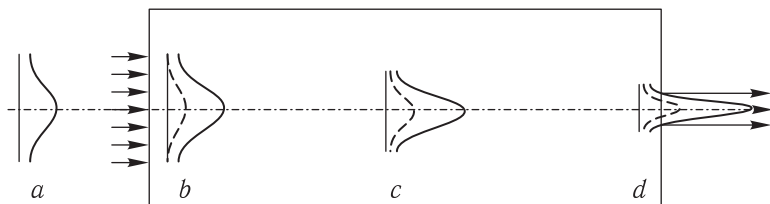
Рис. 185. Распределение интенсивности излучения и показателя преломления по сечению лазерного пучка лучей на входе в кювету ( a ), вблизи входного торца ( b ), в середине кюветы ( c ), вблизи выходного торца кюветы ( d )
