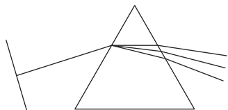
Рис. 190. Разложение белого света при преломлении в призме. Падающий пучок белого света изображен в виде фронта с перпендикулярным к нему направлением распространения волн. Для преломленных пучков показаны только направления распространения волн
