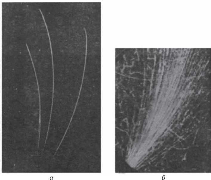
Рис. 380. Следы \alpha - и \beta -частиц в камере Вильсона. Частицы испускаются радиоактивным препаратом, помещенным в нижней части камеры: а) \alpha -частицы: камера в магнитном поле 4,3 Тл, направленном перпендикулярно плоскости рисунка от нас; б) \beta -частицы: магнитное поле 0,0215 Тл направлено на нас
