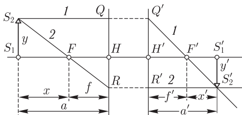
Рис. 226. Построение изображения в оптической системе
