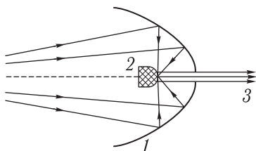
Рис. 169. Схема «гиперболоида»: 1 — собирающее гиперболическое зеркало, 2 — отражающий гиперboloид, 3 — параллельный пучок лучей
