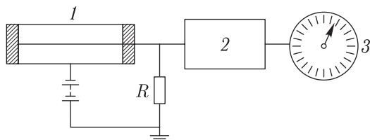
Рис. 384. Схема установки для регистрации радиоактивных излучений с помощью газоразрядного счетчика: 1 — газоразрядный счетчик, 2 — усилитель, 3 — электромагнитный нумератор, R \sim 1 \text{ МОм}
