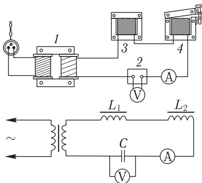
Рис. 53. Получение электрического резонанса на частоту городского тока: 1 — трансформатор, понижающий напряжение, например с 220 до 6 В, 2 — конденсатор емкости C = 1,2 мкФ, 3 — дроссель, индуктивность которого L_1 = 7,5 Гн, а сопротивление обмотки равно 80 Ом, 4 — дроссель с переменным воздушным зазором, индуктивность которого L_2 = 8,3 Гн при ширине зазора 2–3 мм и изменяется при изменении ширины зазора на 15–20 % в обе стороны от указанного (резонансного) значения
