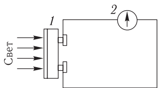
Рис. 153. Фотоэлемент с электрической схемой: 1 — фотоэлемент, 2 — гальванометр
