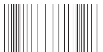
Продольная волна
