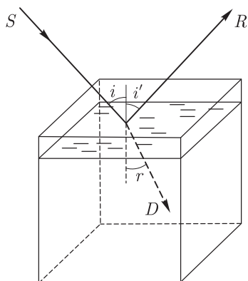
Рис. 180. Преломление и отражение света при падении луча на поверхность воды
