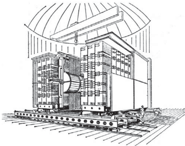
Рис. 422. Общий вид экспериментальной установки UA-1, на которой проводились исследования \bar{p}p -соударений на самом большом в мире ускорителе-накопителе со встречными протонным и антипротонным пучками (SPS-коллайдер ЦЕРН, см. табл. 12). Установка UA-1 — это огромный магнитный спектрометр для измерения импульсов вторичных частиц, образующихся в \bar{p}p -соударениях. Частицы регистрировались в газоразрядной камере (она видна в центре установки). Камера представляет собой совокупность большого числа газоразрядных детекторов частиц, напоминающих пропорциональные счетчики. С помощью этих детекторов определяются траектории частиц. В состав установки входит также большое число сцинтилляционных счетчиков
