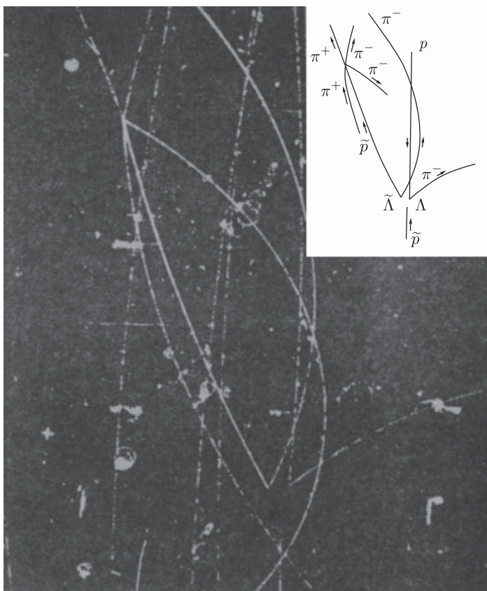
Рис. 419. Образование и распад \Lambda -гиперонов. В водородной пузырьковой камере, находившейся в магнитном поле и облученной антипротонами, зафиксирована реакция \tilde{p} + p \rightarrow \tilde{\Lambda} + \Lambda . Она произошла в точке окончания следа \tilde{p} (см. схему в верхней части рисунка). Нейтральные лямбда- и антилямбда-гипероны, пролетев без образования следа небольшой путь, распадаются по схемам \Lambda \rightarrow p + \pi^- , \tilde{\Lambda} \rightarrow \tilde{p} + \pi^+ . Антипротон \tilde{p} аннигилирует с протоном, образуя два \pi^+ - и два \pi^- -мезона
