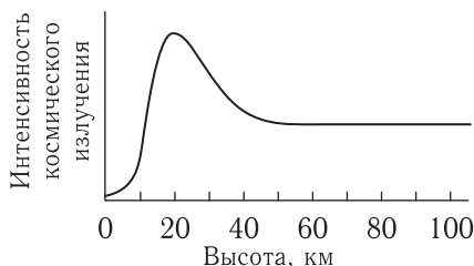
Рис. 421. Зависимость интенсивности космического излучения от высоты над уровнем моря. На высотах выше 50 км присутствует только первичная компонента космического излучения, приходящая из мирового пространства, и интенсивность излучения не зависит от высоты. Ниже 50 км интенсивность вначале увеличивается за счет образования вторичных частиц, а затем падает за счет возрастающего поглощения в атмосфере
