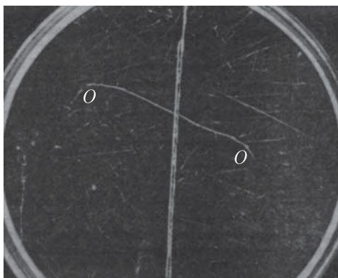
Рис. 403. Фотография следов осколков деления урана в камере Вильсона: осколки (O) разлетаются в противоположные стороны из тонкого слоя урана, нанесенного на пластинке, перегородивающей камеру. На снимке видно также множество более тонких следов, принадлежащих протонам, выбитым нейтронами из молекул водяного пара, содержащегося в камере
