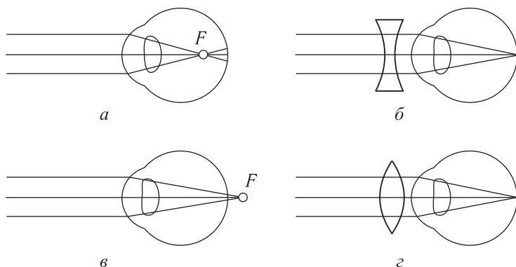
Рис. 247. Близорукость глаза (а) исправляется с помощью рассеивающей линзы (б); дальность зрения (в) — с помощью собирающей линзы (г)
