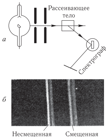
Рис. 371. а) Схема опыта Комптона. б) Спектр рассеянного рентгеновского излучения
