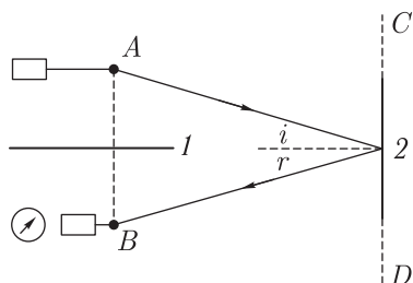
Рис. 128. Отражение электромагнитной волны: i — угол падения, r — угол отражения
