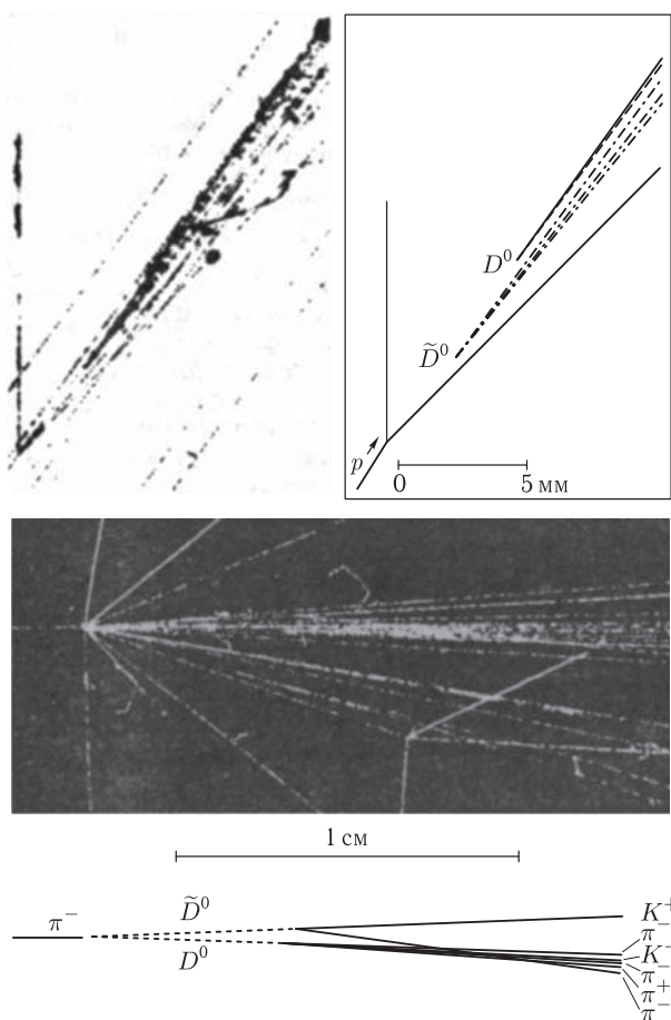
Рис. 424. Образование и распад очарованных D^0 и \bar{D}^0 -мезонов. На рисунке показаны две фотографии событий парного образования очарованных частиц в реакции \pi^- + p \rightarrow D^0 + \bar{D}^0 (другие частицы) в пузырьковых камерах с высоким пространственным разрешением. D^0 -мезоны имеют время жизни \sim 10^{-12} с и пролетают расстояния в несколько мм. Зарегистрированы их распады D^0 \rightarrow K^- + \pi^+ + \pi^+ + \pi^- и \bar{D}^0 \rightarrow K^+ + \pi^- . Вверху справа и внизу приведены схемы соответствующих событий
