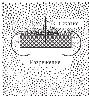
Рис. 109. Вид на ножку камертона сверху. Жирной стрелкой показано направление ее движения, а тонкими стрелками — распространение волны сжатия вокруг ножки
