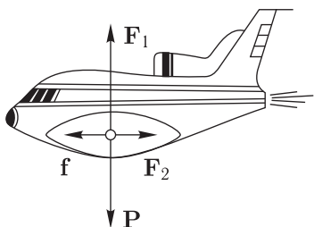
Рис. 348. Силы, действующие на самолет при горизонтальном равномерном полете
