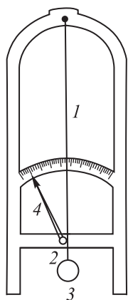
Рис. 503. Волосной гигрометр
