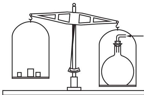
Рис. 273. Взвешивание воздуха
