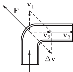
Рис. 319. При изменении направления течения воды на трубку действует сила реакции струи воды \mathbf{F}
