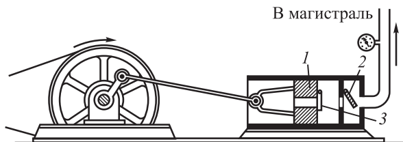
Рис. 302. Схема компрессора
