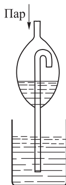
Рис. 489. Сухопарник — приспособление для задержания капелек воды, движущихся вместе с паром
