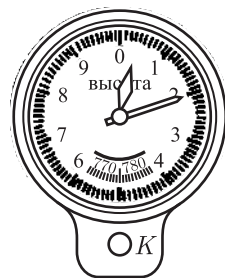
Рис. 295. Самолетный альтиметр. Длинная стрелка отсчитывает сотни метров, короткая — километры. Головка K позволяет подводить ноль циферблата под стрелку на поверхности Земли перед началом полета
