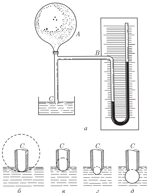
Рис. 419. a ) Прибор для выдувания пузырьков в жидкости. б )– г ) В начале выдувания пузырька радиус кривой поверхности жидкости постепенно уменьшается. д ) Под конец выдувания радиус поверхности снова увеличивается
