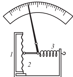
Рис. 293. Схема устройства мембранного манометра для газов
