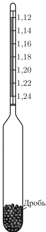
Рис. 266. Ареометр (шкала в 10^3 \text{ кг/м}^3 )
