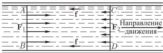
Рис. 309. Сумма сил давления \mathbf{F}_1 и \mathbf{F}_2 уравнивает силы трения \mathbf{f} со стороны стенок трубы
