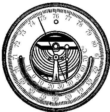
Рис. 294. Барометр-анероид
