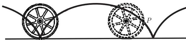
Рис. 5. Точка P на ободе катящегося колеса описывает относительно земной поверхности траекторию, изображенную на рисунке (циклоиду)
