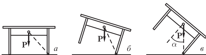
Рис. 134. При отклонении стола ( b ) от его положения равновесия ( a ) центр тяжести поднимается — равновесие устойчиво. В положении v ) стол отклонен на предельный угол; при дальнейшем отклонении центр тяжести будет опускаться — равновесие неустойчиво
