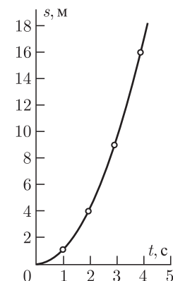
Рис. 37. График пути при равноускоренном движении
