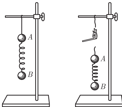
Рис. 86. При пережигании нити шарик A движется с ускорением, большим g , а шарик B — с ускорением, меньшим g , и шарiki сближаются; деформация пружины исчезает
