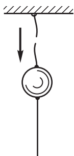
Рис. 87. Если медленно тягивать нижнюю нить, то оборвется верхняя нить
