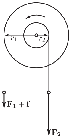
Рис. 156. Увеличив силу F_1 на малую величину f , заставим блок вращаться с ускорением
