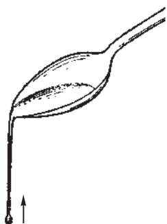
Рис. 399. Струйка меда, стекающая с ложки, собирается в шарик, поднимающийся вверх
