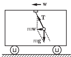
Рис. 205. Отклонение отвеса в ускоренно движущемся вагоне
