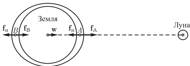
Рис. 211. Возникновение приливов: f_{\text{и}} — сила инерции, f_A и f_B — силы притяжения частиц воды Луной, w — ускорение Земли, вызванное притяжением Луны
