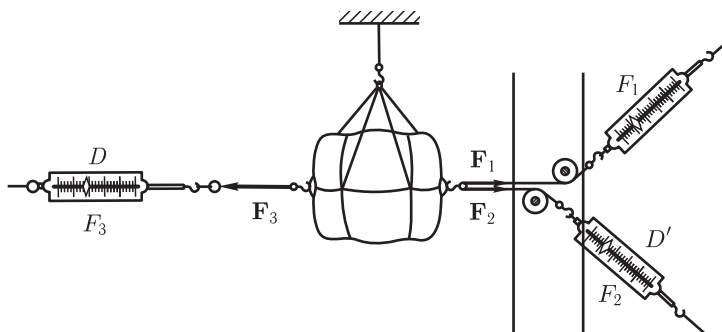
Рис. 63. Показание динамометра D дает модуль равнодействующей сил \mathbf{F}_1 и \mathbf{F}_2 . Показание динамометра D' дает модуль равнодействующей сил \mathbf{F}_1 и \mathbf{F}_3
