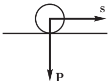
Рис. 157. При качении шара по горизонтальному столу сила тяжести \mathbf{P} перпендикулярна к перемещению \mathbf{s} и ее работа равна нулю
