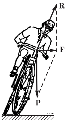
Рис. 194. Велосипедист наклоняется в сторону поворота. Сила тяжести \mathbf{P} и сила реакции \mathbf{R} со стороны земли дают равнодействующую силу \mathbf{F} , сообщающую центростремительное ускорение, необходимое для движения по окружности
