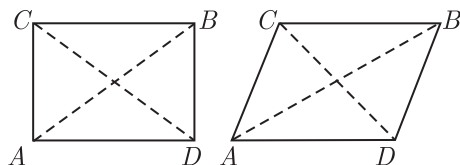
Рис. 463. Сдвиг сопровождается удлинением по направлению AB и укорочением по направлению CD
