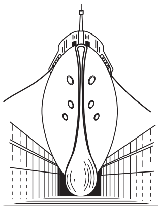
Рис. 338. «Бульбообразный» нос быстроходного судна
