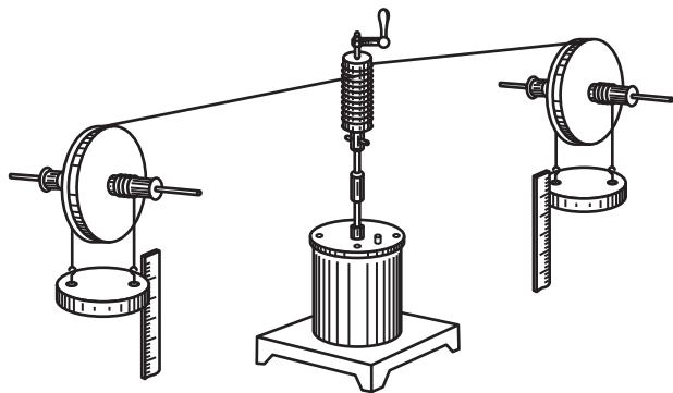
Рис. 365. Прибор Джоуля
