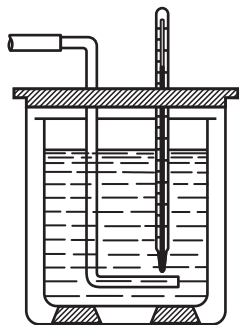
Рис. 367. Калориметр
