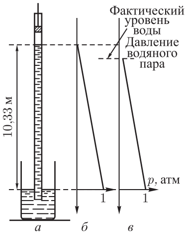
Рис. 289. а) То же, что на рис. 288, но при поднятии поршня выше предельной высоты (10,33 м). б) График давления для такого положения поршня. в) В действительности столб воды не достигает полной высоты, так как водяной пар имеет при комнатной температуре давление около 20 мм рт. ст. и соответственно понижает верхний уровень столба. Поэтому истинный график имеет срезанную верхушку. Для наглядности давление водяного пара преувеличено
