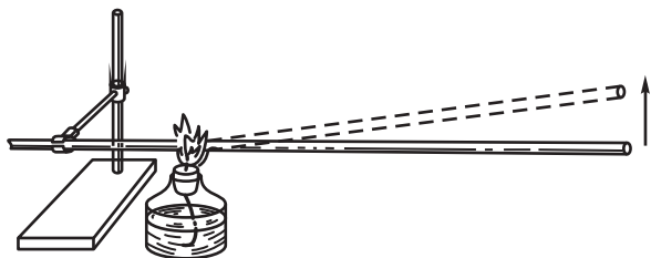
Рис. 354. Стеклянная трубка при нагревании ее снизу заметно изгибается вверх
