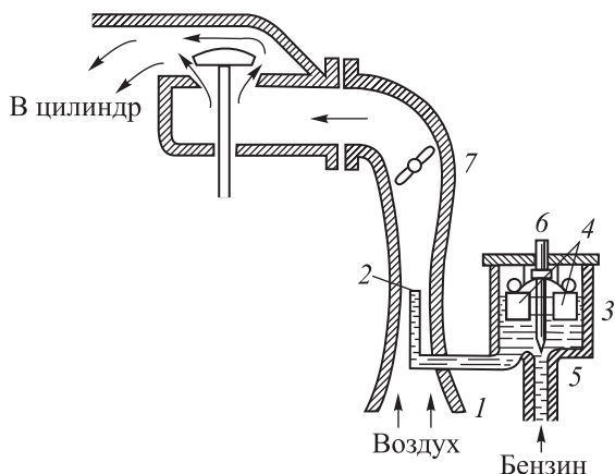
Рис. 523. Устройство карбюратора
