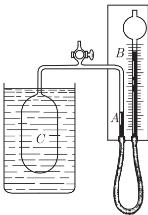
Рис. 386. Газовый термометр
