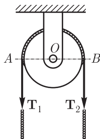
Рис. 140. Простой блок
