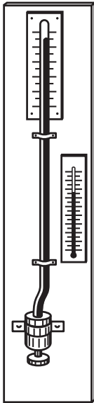
Рис. 291. Ртутный барометр
