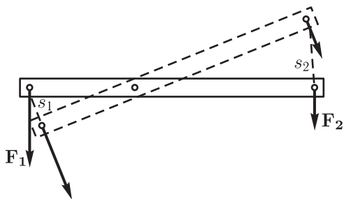
Рис. 155. Сила, действующая на левое плечо рычага, в n раз больше силы, действующей на правое плечо. Путь s_1 , пройденный точкой приложения силы \mathbf{F}_1 , будет в n раз меньше пути s_2 , пройденного точкой приложения силы \mathbf{F}_2
