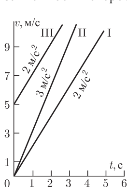
Рис. 30. Графики скорости различных равноускоренных движений
