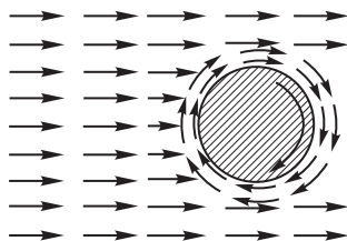
Рис. 342. При вращении цилиндра скорость увлекаемого воздуха с одной стороны складывается со скоростью потока (вверх), а с другой — вычитается (вниз)
