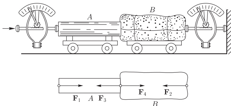
Рис. 69. Исследование взаимодействия двух тел A и B . Внизу показаны действующие на них силы
