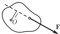
Рис. 115. Момент силы \mathbf{F} равен произведению ее модуля F на плечо l
