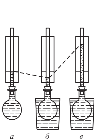
Рис. 357. а ) Подкрашенная вода вошла из колбы в пробку. б ) К колбе снизу подносится сосуд с горячей водой. В первый момент погружения колбы жидкость в трубке опускается. в ) Уровень в трубке через некоторое время устанавливается выше, чем до нагревания колбы
