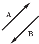
Рис. 40. Векторы различаются только знаком: \mathbf{A} = -\mathbf{B}
