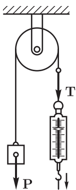
Рис. 94. Чтобы груз поднимался, сила T должна быть больше силы тяжести P , действующей на груз
