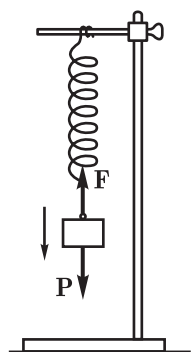
Рис. 159. При опускании груза работа силы \mathbf{P} положительна, а силы \mathbf{F} отрицательна
