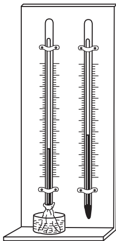
Рис. 504. Психрометр
